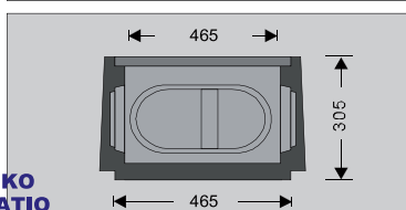
ΠΡΟΕΚΤΑΣΗ ΦΡΕΑΤΙΟΥ
